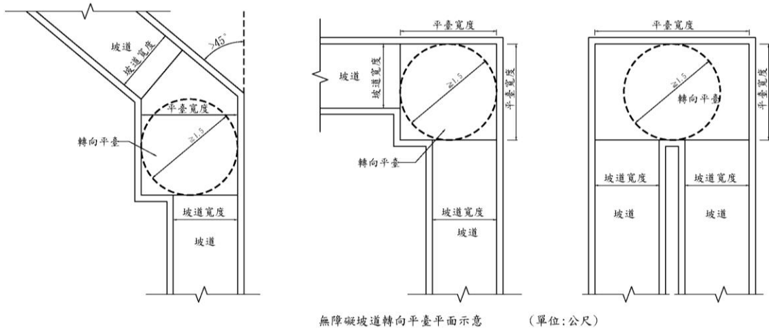
無障礙坡道及平臺參考圖
